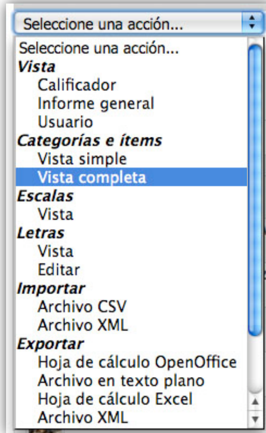
Figura 2. Menú desplegable
