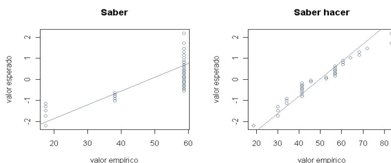
Gráfico 5.26 Gráficos Q-Q normales postest. Aspectos básicos.
