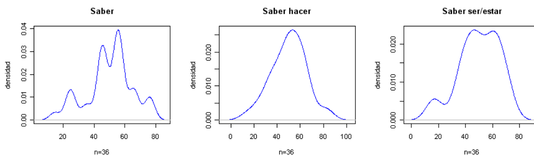
Gráfico 5.18 Funciones de densidad posttest. Búsqueda de información.
