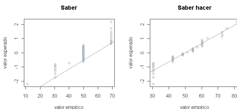
Gráfico 5.11 Gráficos Q-Q normales pretest. Aspectos básicos.
