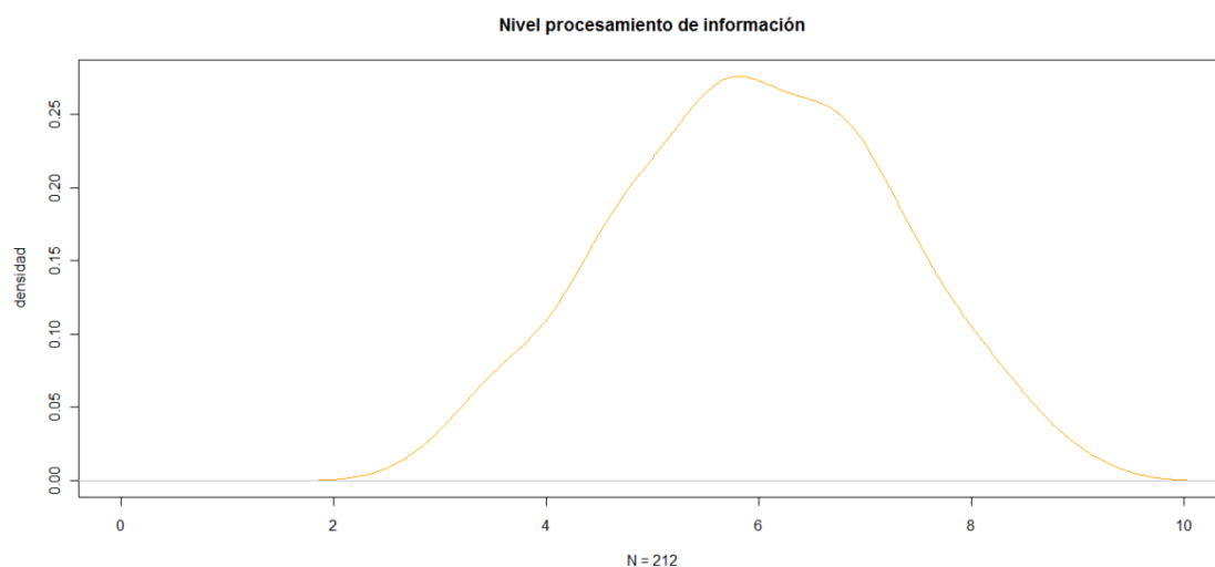
Gráfico 4.44 Función de densidad del nivel autopercibido en el procesamiento de información. Futuro profesorado
