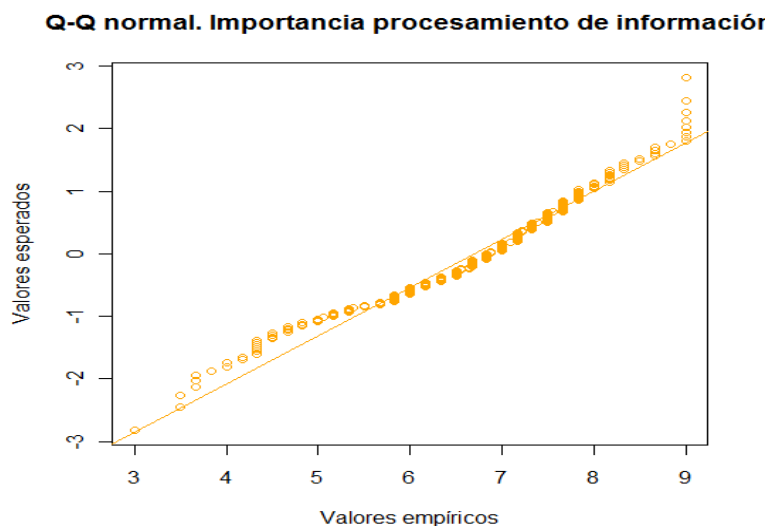
Gráfico 4.40 Q-Q normal para la importancia en el procesamiento de información. Futuro profesorado
