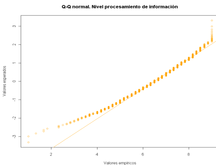
Gráfico 4.23 Q-Q normal para el nivel autopercebido en el procesamiento de información. Alumnos
