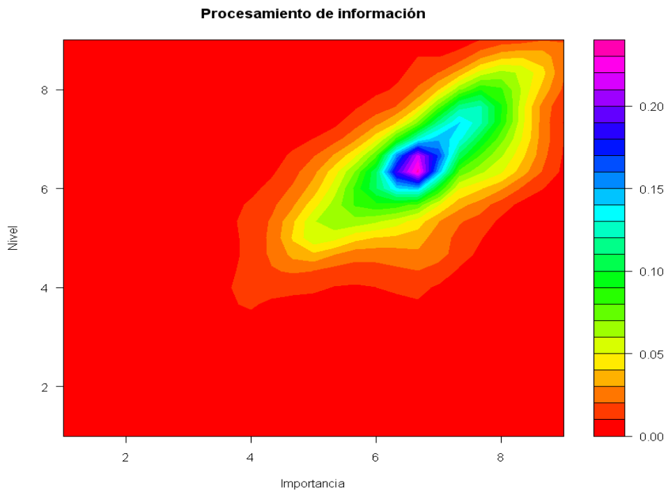
Gráfico 4.27 Distribución de densidad conjunta para el nivel y la importancia en el procesamiento. Alumnos
