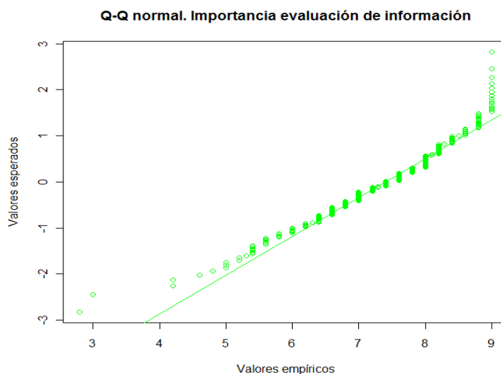
Gráfico 4.39 Q-Q normal para la importancia en la evaluación de información. Futuro profesorado
