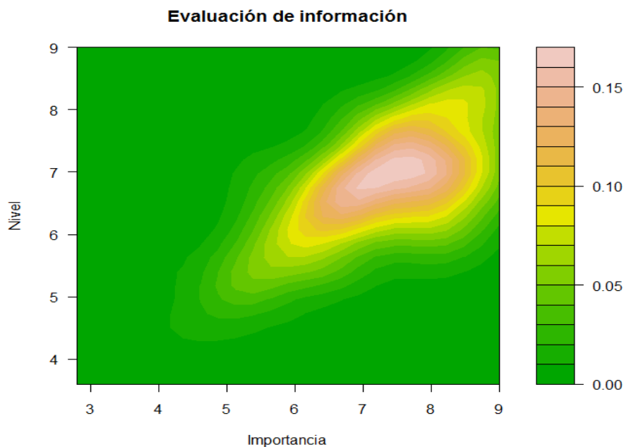
Gráfico 4.52 Distribución de densidad conjunta para el nivel y la importancia en la evaluación. Futuro profesorado
