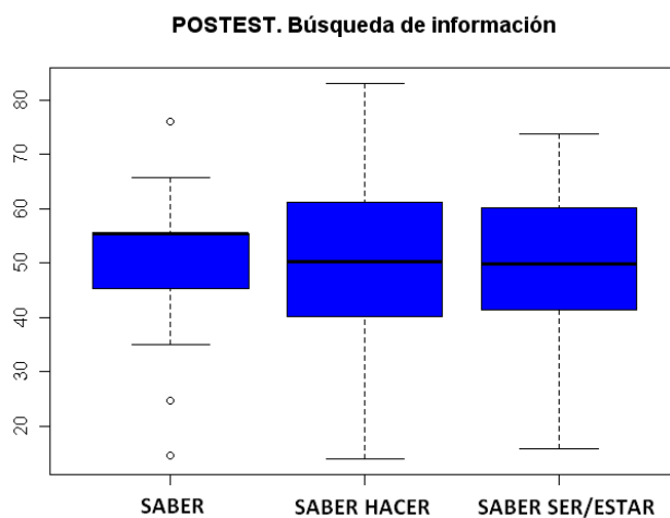
Gráfico 5.19 Diagramas de cajas postest. Búsqueda de información.
