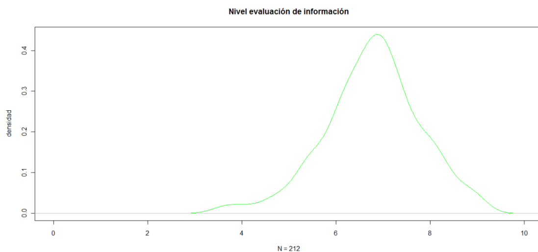
Gráfico 4.43 Función de densidad del nivel autopercibido en la evaluación de información. Futuro profesorado
