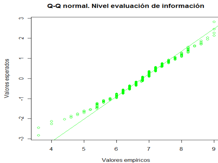
Gráfico 4.48 Q-Q normal para el nivel autopercibido en la evaluación de información. Futuro profesorado
