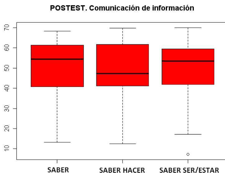
Gráfico 5.25 Diagramas de cajas posttest. Comunicación de información.
