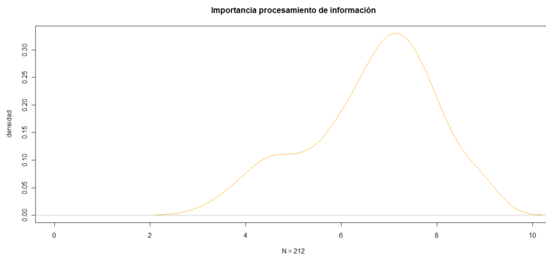
Gráfico 4.35 Función de densidad de la importancia asignada al procesamiento de información. Futuro profesorado
