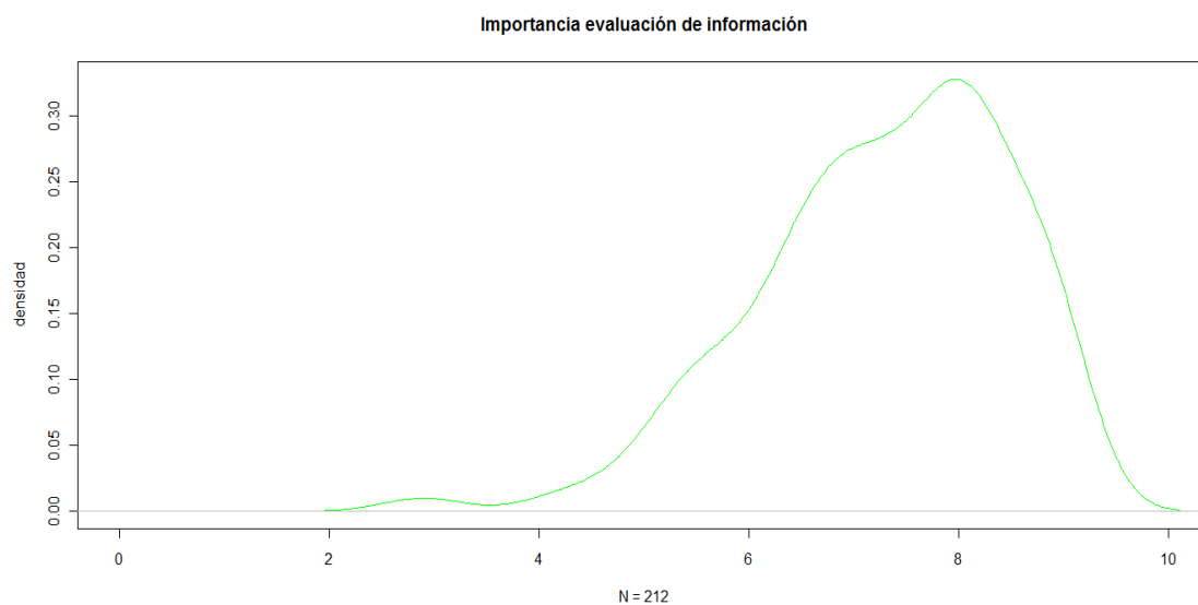
Gráfico 4.34 Función de densidad de la importancia asignada a la evaluación de información. Futuro profesorado
