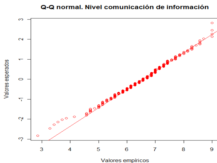
Gráfico 4.50 Q-Q normal para el nivel autopercebido en la comunicación de información. Futuro profesorado
