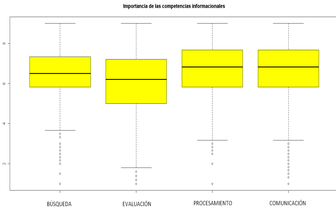
Gráfico 4.11 Diagramas de cajas importancia percibida sobre competencias informacionales. Alumnos
