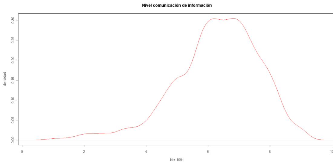
Gráfico 4.19 Función de densidad del nivel autopercebido en la comunicación de información. Alumnos
