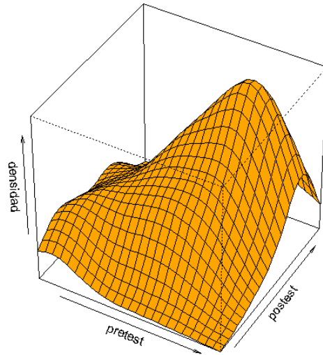
Gráfico 5.34 Funciones de densidad conjuntas evaluación y tratamiento. Saber hacer
