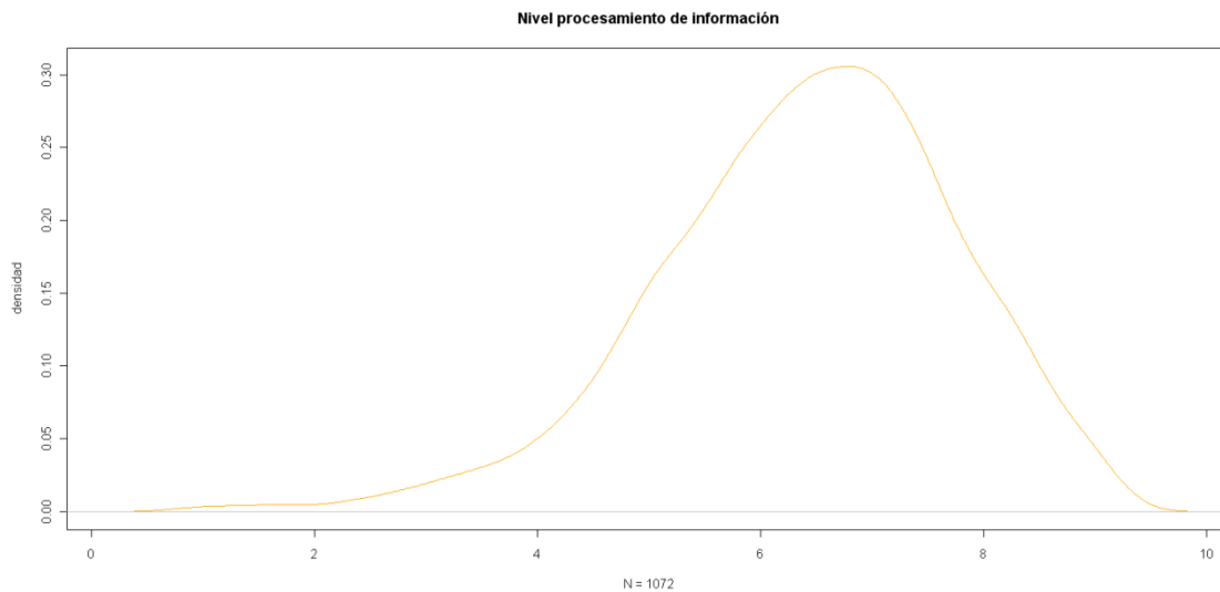
Gráfico 4.18 Función de densidad del nivel autopercebido en el procesamiento de información. Alumnos
