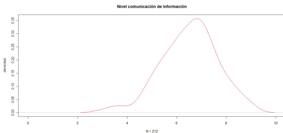
Gráfico 4.45 Función de densidad del nivel autopercibido en la comunicación de información. Futuro profesorado
