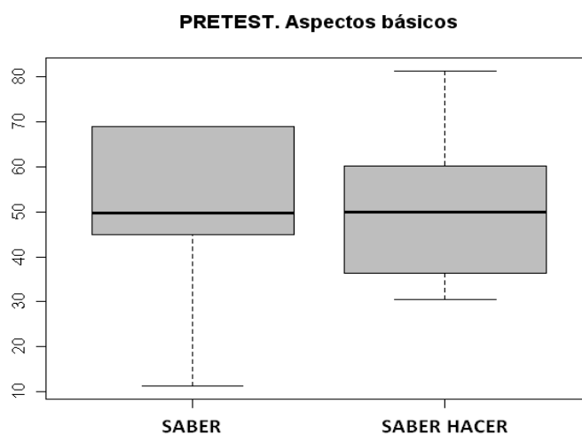
Gráfico 5.2 Diagramas de cajas pretest. Aspectos básicos.
