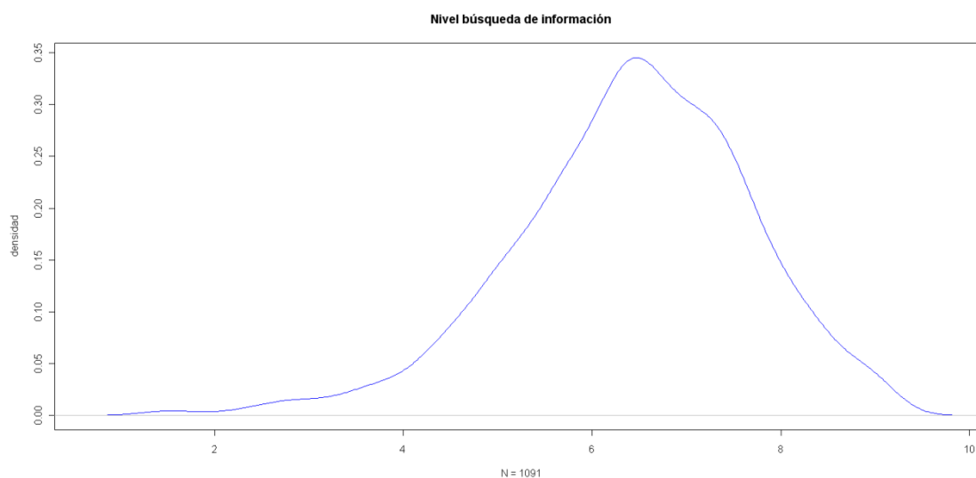
Gráfico 4.16 Función de densidad del nivel autopercebido en la búsqueda de información. Alumnos
