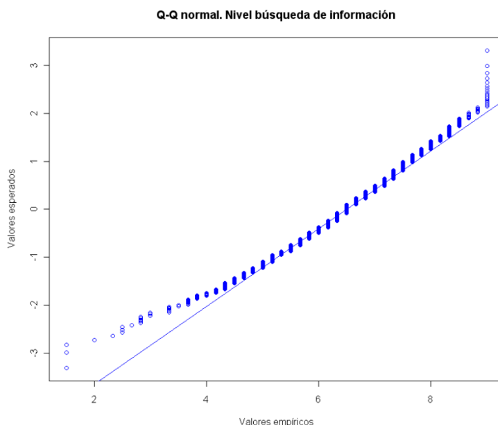
Gráfico 4.21 Q-Q normal para el nivel autopercebido en la búsqueda de información. Alumnos
