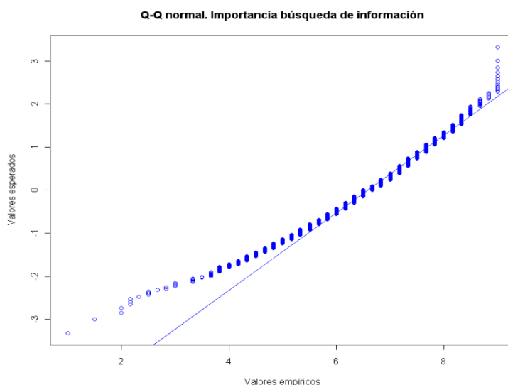
Gráfico 4.12 Q-Q normal para la importancia en la búsqueda de información. Alumnos
