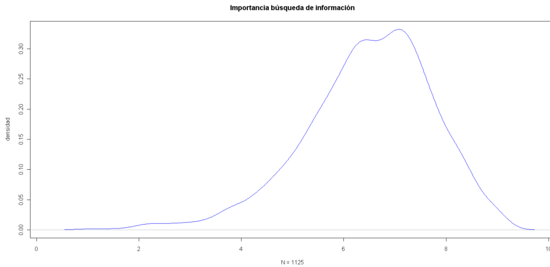
Gráfico 4.7 Función de densidad de la importancia asignada a la búsqueda de información. Alumnos
