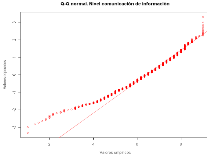
Gráfico 4.24 Q-Q normal para el nivel autopercebido en la comunicación de información. Alumnos
