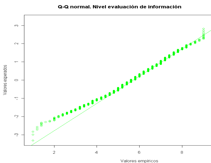
Gráfico 4.22 Q-Q normal para el nivel autopercebido en la evaluación de información. Alumnos
