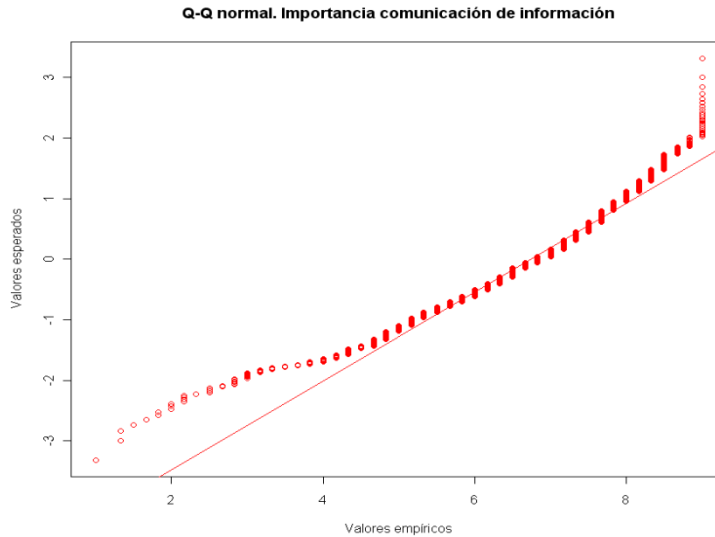
Gráfico 4.15 Q-Q normal para la importancia en la comunicación de información. Alumnos
