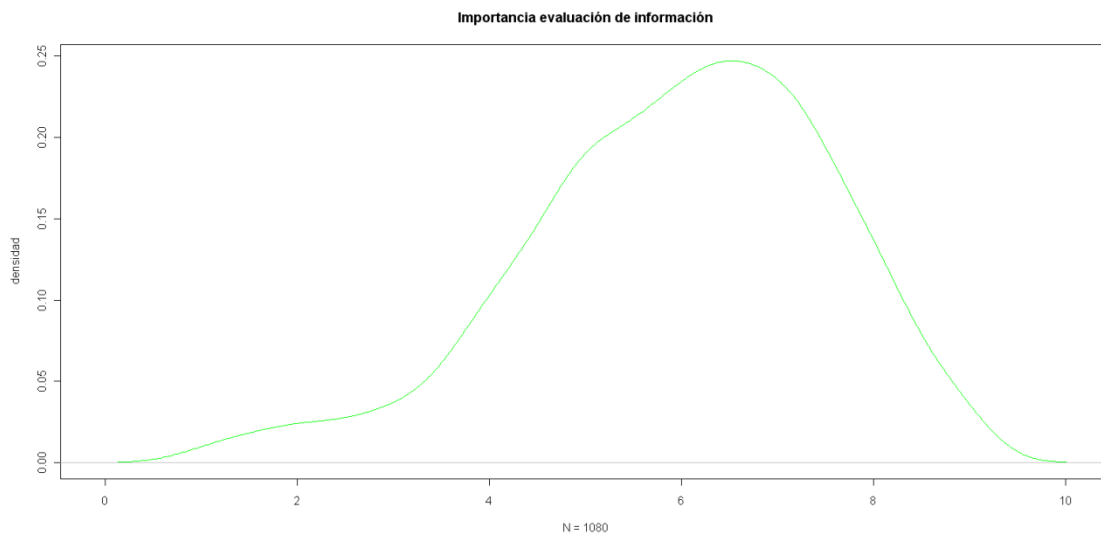
Gráfico 4.8 Función de densidad de la importancia asignada a la evaluación de información. Alumnos
