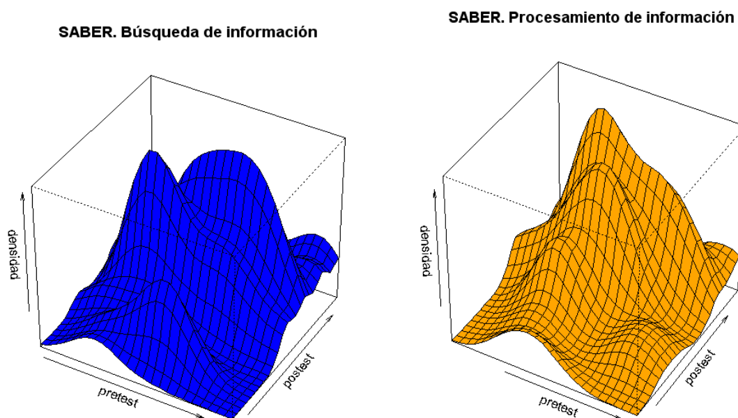
Gráfico 5.32 Funciones de densidad conjuntas búsqueda y procesamiento. Saber
