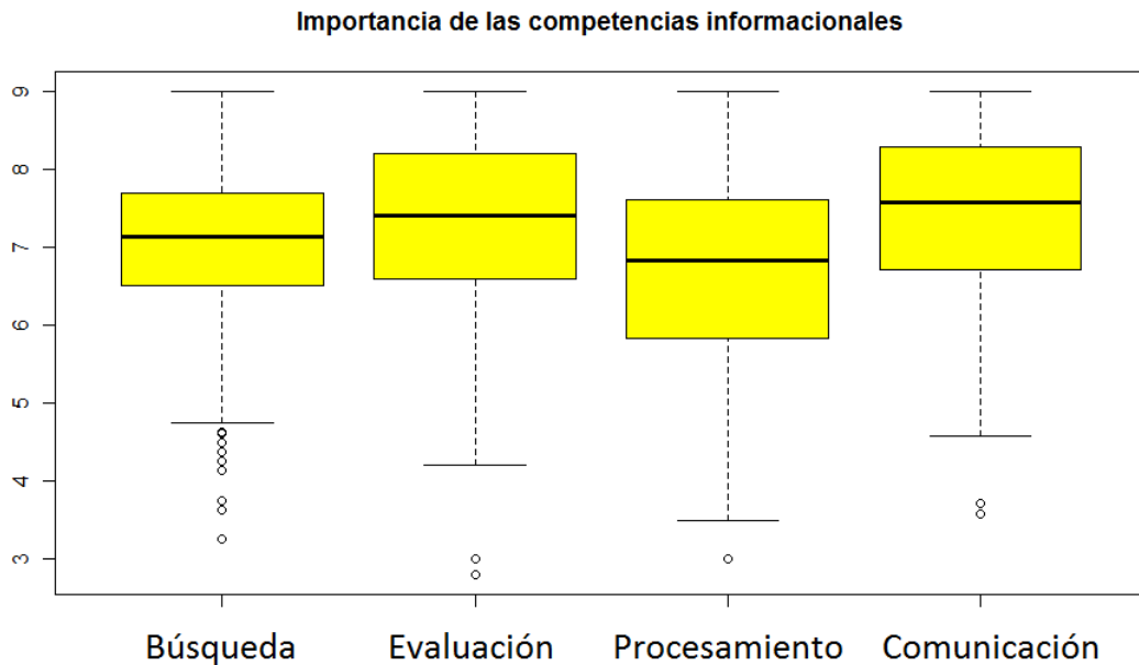
Gráfico 4.37 Diagramas de cajas importancia percibida sobre competencias informacionales. Futuro profesorado
