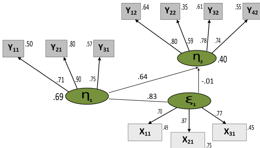
Figura 4.19 Solución estandarizada del modelo planteado. Futuro profesorado
