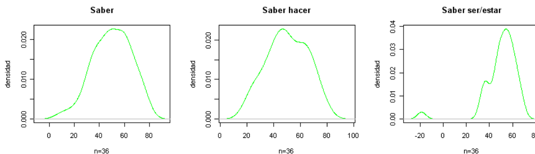
Gráfico 5.5 Funciones de densidad pretest. Evaluación de información.
