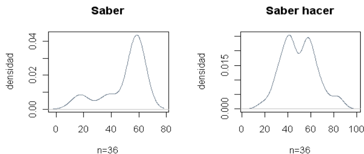
Gráfico 5.16 Funciones de densidad postest. Aspectos básicos.
