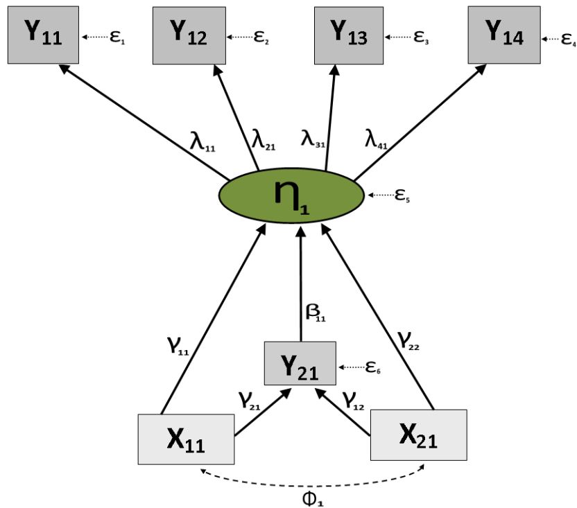
Figura 4.13 Diseño del modelo de ecuaciones estructurales teórico. Alumnos
