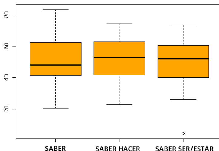
Gráfico 5.8 Diagramas de cajas pretest. Procesamiento de información.
