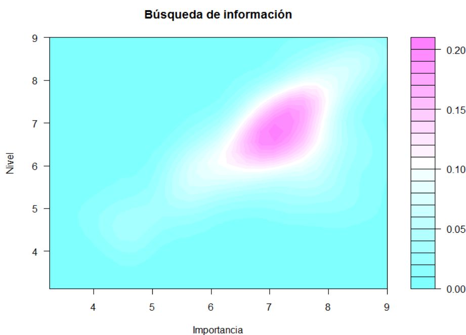
Gráfico 4.51 Distribución de densidad conjunta para el nivel y la importancia en la búsqueda. Futuro profesorado
