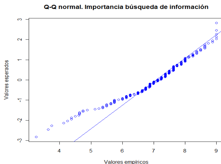
Gráfico 4.38 Q-Q normal para la importancia en la búsqueda de información. Futuro profesorado
