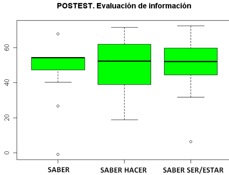
Gráfico 5.21 Diagramas de cajas posttest. Procesamiento de información.
