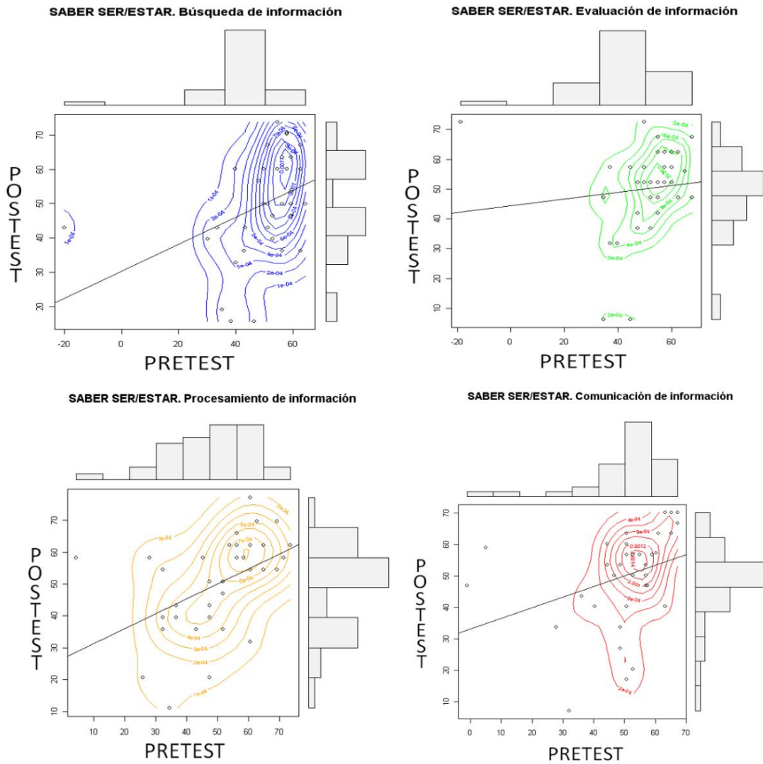
Gráfico 5.35 Diagramas de dispersión e histograma variables bidimensionales. Saber ser/estar
