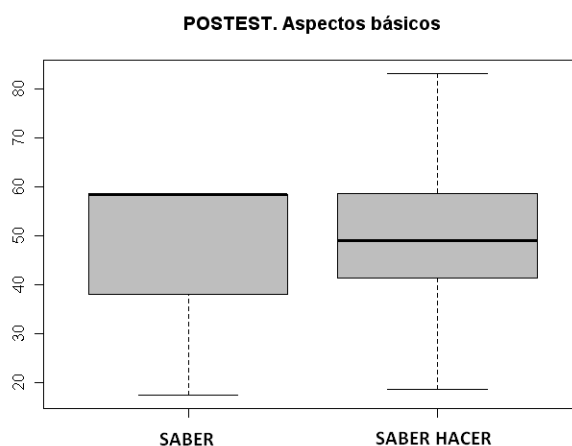
Gráfico 5.17 Diagramas de cajas posttest. Aspectos básicos.
