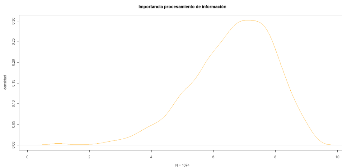
Gráfico 4.9 Función de densidad de la importancia asignada al procesamiento de información. Alumnos
