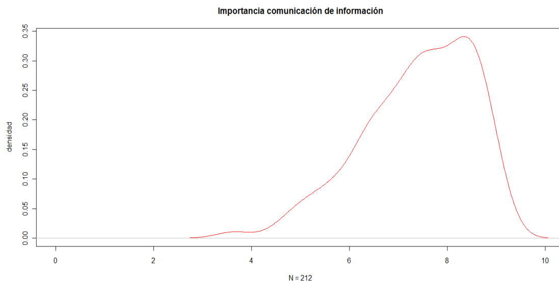
Gráfico 4.36 Función de densidad de la importancia asignada a la comunicación de información. Futuro profesorado
