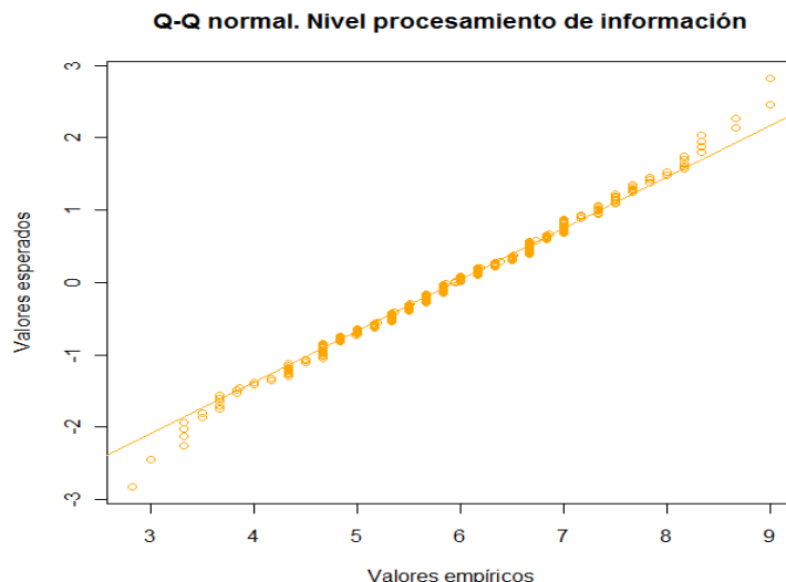
Gráfico 4.49 Q-Q normal para el nivel autopercebido en el procesamiento de información. Futuro profesorado
