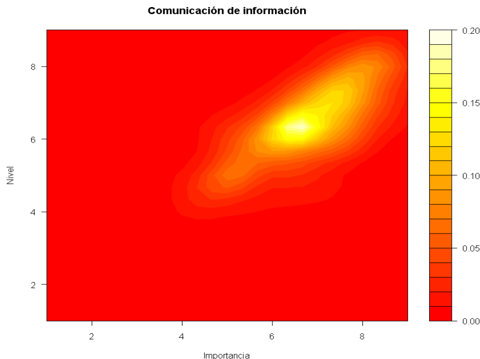
Gráfico 4.28 Distribución de densidad conjunta para el nivel y la importancia en la comunicación. Alumnos
