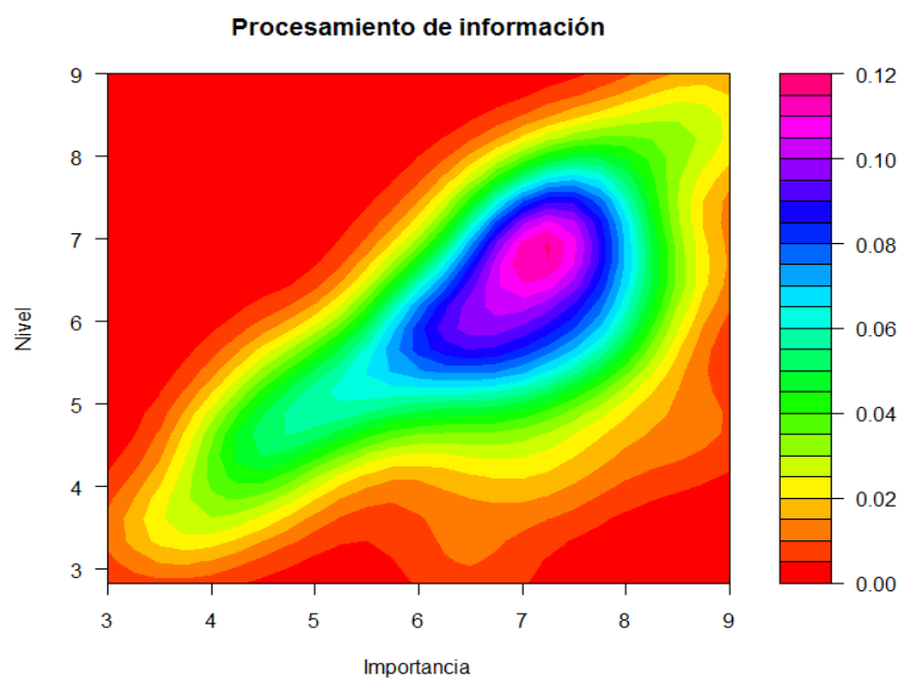
Gráfico 4.53 Distribución de densidad conjunta para el nivel y la importancia en el procesamiento. Futuro profesorado
