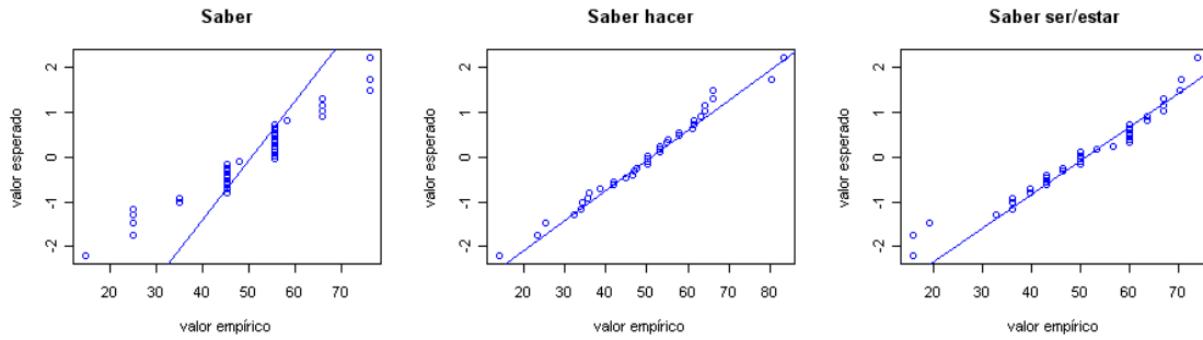
Gráfico 5.27 Gráficos Q-Q normales posttest. Búsqueda de información.
