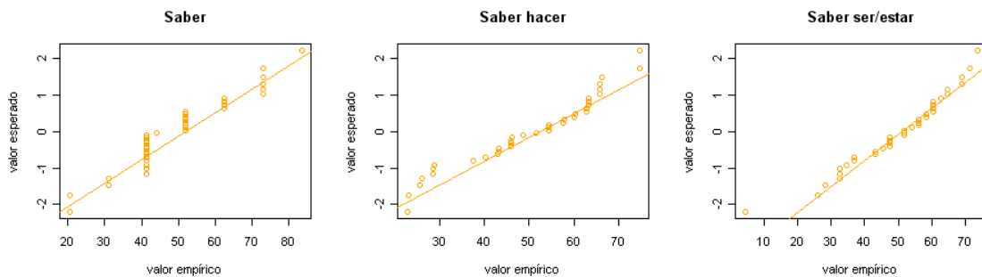
Gráfico 5.14 Gráficos Q-Q normales pretest. Procesamiento de información.
