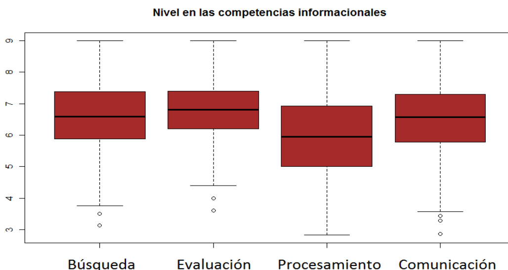
Gráfico 4.46 Diagramas de cajas nivel autopercebido sobre competencias informacionales. Futuro profesorado
