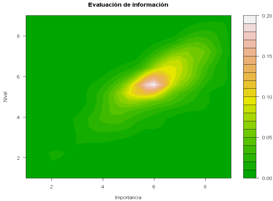
Gráfico 4.26 Distribución de densidad conjunta para el nivel y la importancia en la evaluación. Alumnos
