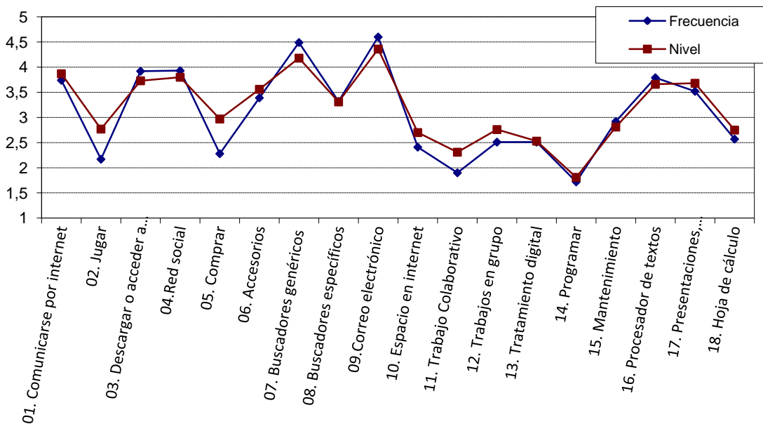
Gráfico 4.31 Diferencias entre la frecuencia y nivel declarados en el manejo de herramientas
