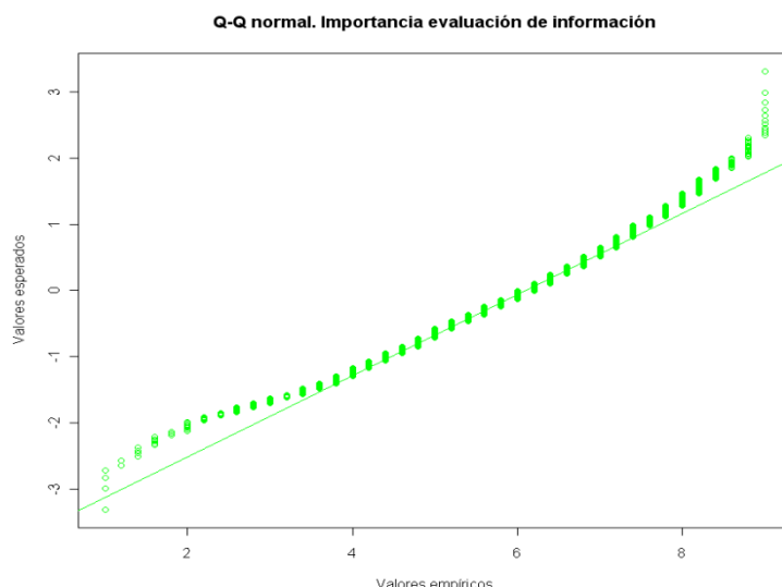
Gráfico 4.13 Q-Q normal para la importancia en la evaluación de información. Alumnos
