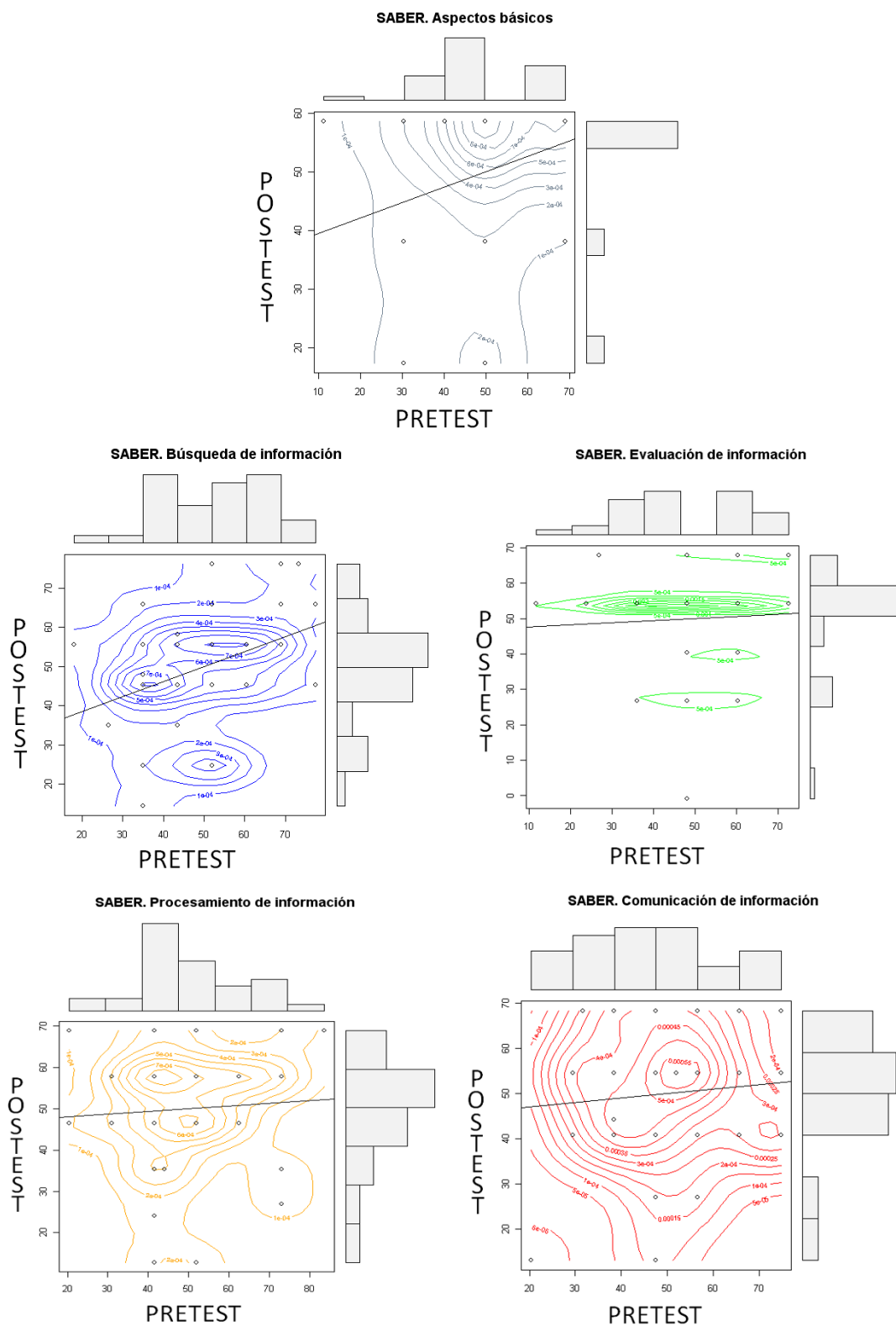
Gráfico 5.31 Diagramas de dispersión e histograma variables bidimensionales. Saber
