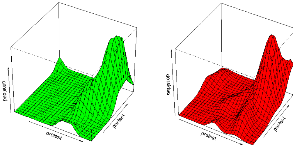
Gráfico 5.36 Funciones de densidad conjuntas evaluación y comunicación. Saber ser/estar
