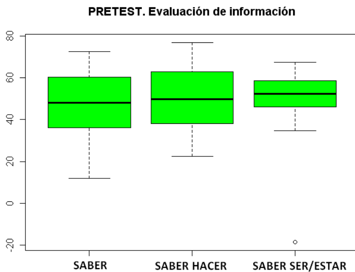
Gráfico 5.6 Diagramas de cajas pretest. Procesamiento de información.
