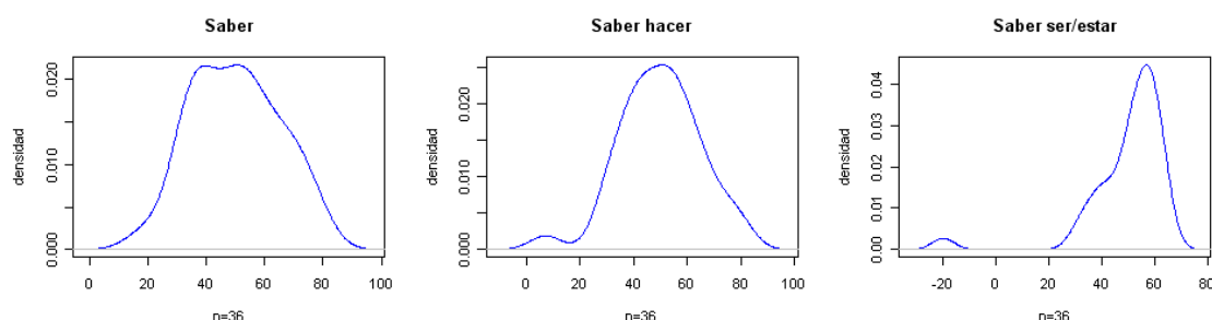
Gráfico 5.3 Funciones de densidad pretest. Búsqueda de información.
