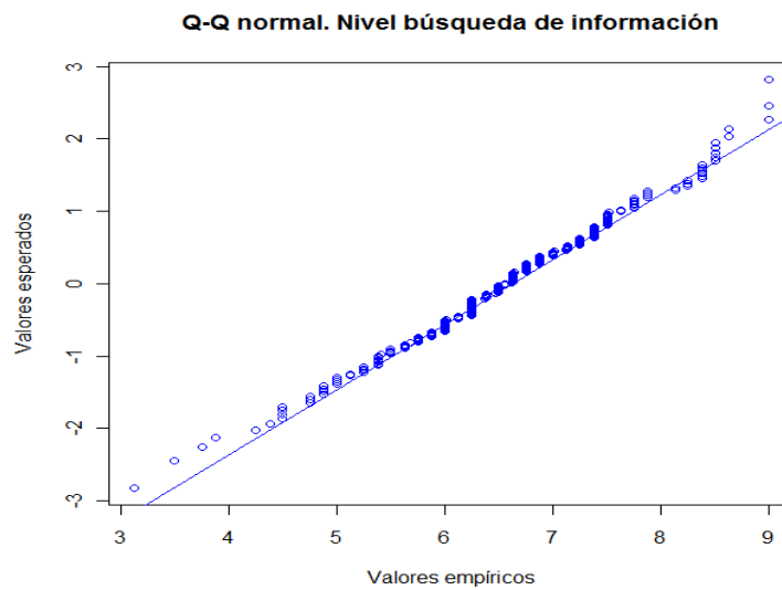
Gráfico 4.47 Q-Q normal para el nivel autopercibido en la búsqueda de información. Futuro profesorado
