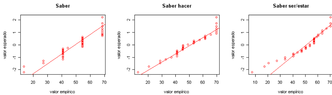
Gráfico 5.30 Gráficos Q-Q normales posttest. Procesamiento de información.
