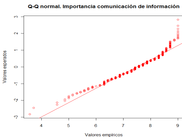
Gráfico 4.41 Q-Q normal para la importancia en la comunicación de información. Futuro profesorado
