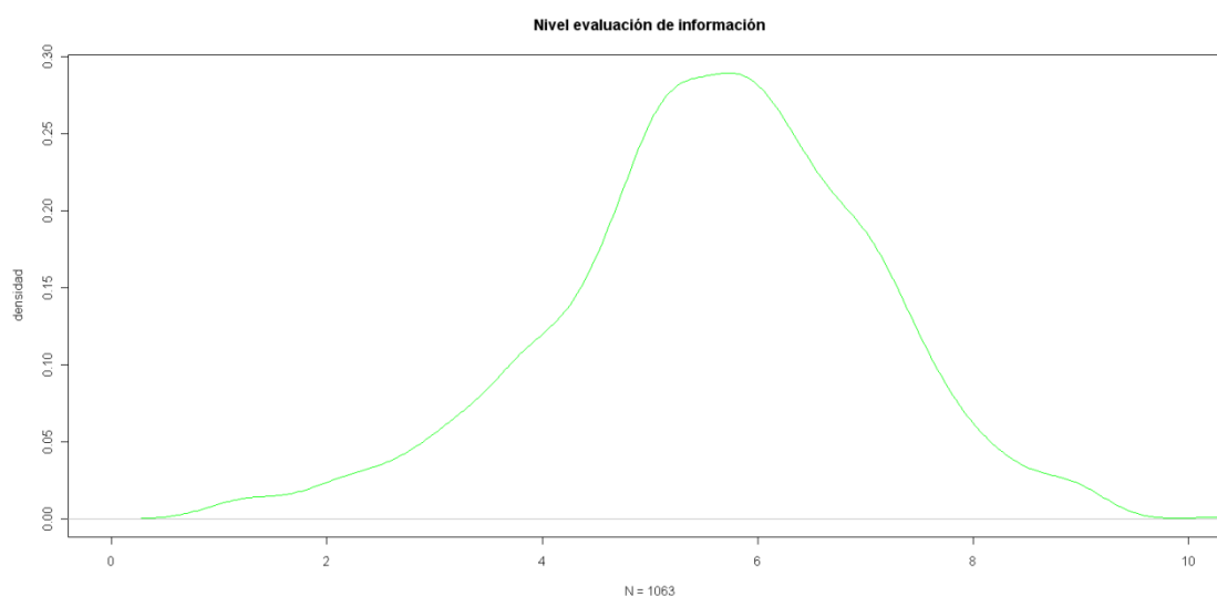
Gráfico 4.17 Función de densidad del nivel autopercebido en la evaluación de información. Alumnos
