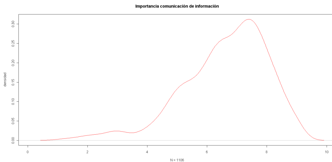
Gráfico 4.10 Función de densidad de la importancia asignada a la comunicación de información. Alumnos
