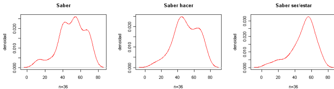
Gráfico 5.24 Funciones de densidad posttest. Comunicación de información.
