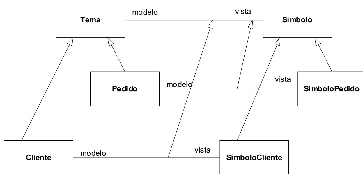
Relaciones de generalización entre asociaciones
