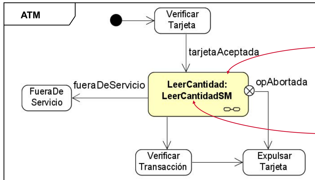
Máquina de estado con el estado de submáquina "LeerCantidad"
