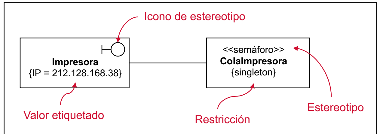
Ejemplos de uso de los mecanismos de extensión
