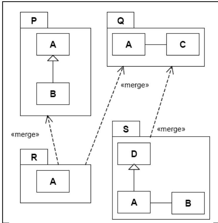
Ejemplo de relaciones <<merge>> entre paquetes
