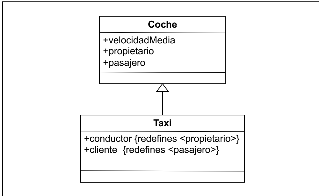
Ejemplos de redefinición de propiedades
