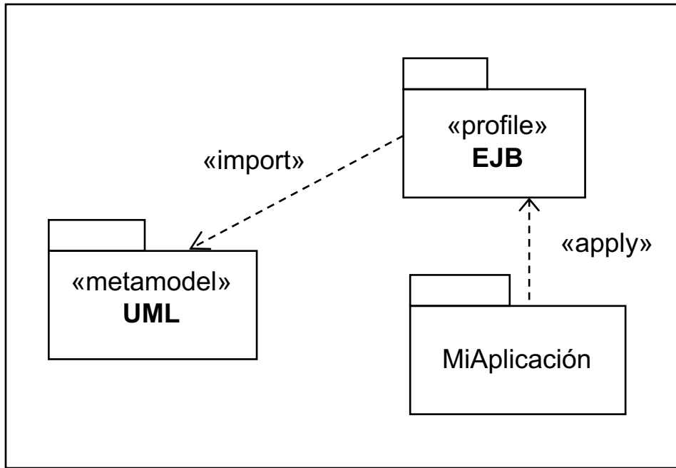
Aplicación del perfil EJB que usa el metamodelo de referencia UML
