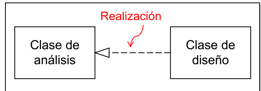
Ejemplos de relaciones de realización
