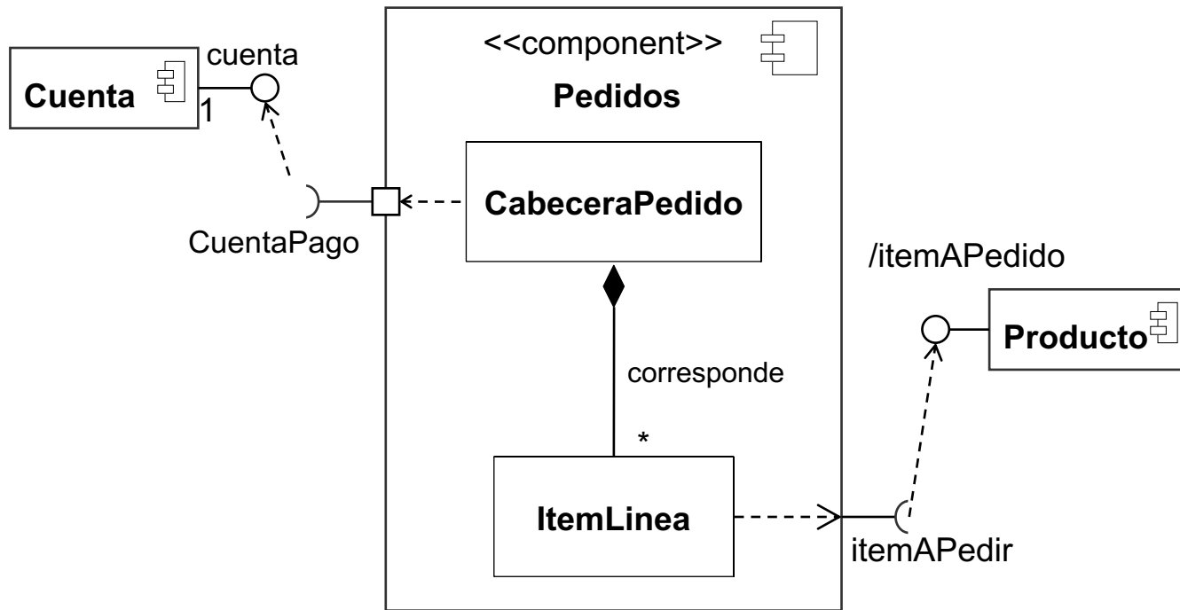
Diagrama de estructura de componentes con interfaces
