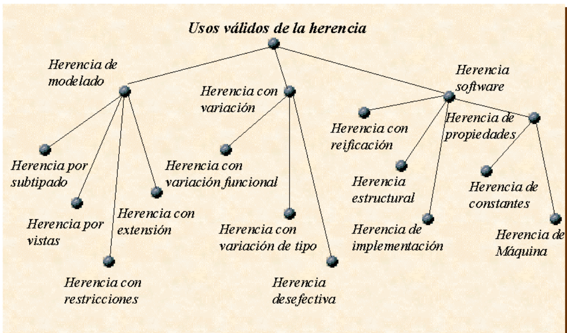
Figura I. Taxonomía de la herencia de Bertrand Meyer.
